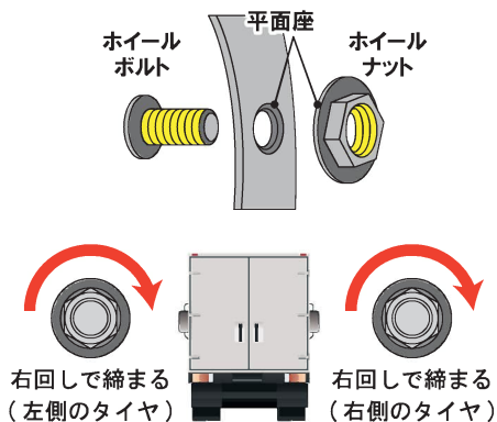
【変更後】ISO 規格（平面座）
