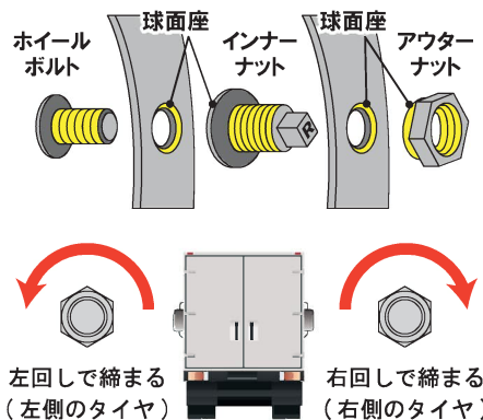
【変更前】JIS 規格（球面座）
